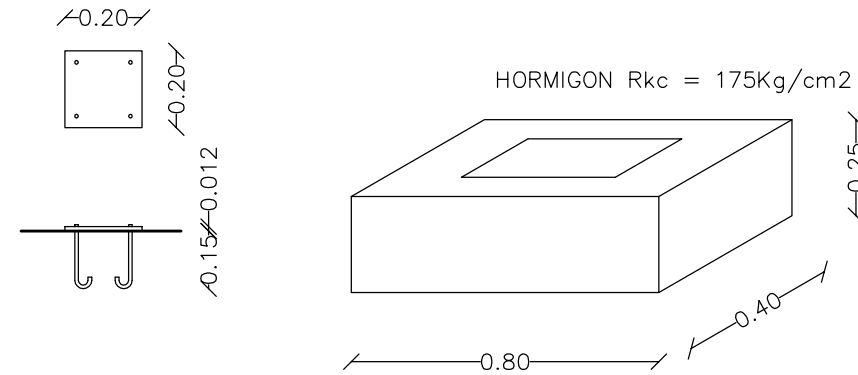
ANCLAJE PILARES PREFABRICADOS DETALLE E: 1/20
