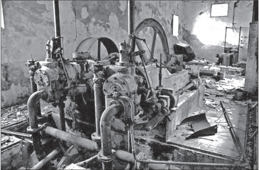
Màquina de vapor que movia l'alternador que donava llum a la mina. Foto cedida per Manuel Espinosa Castellanos.
